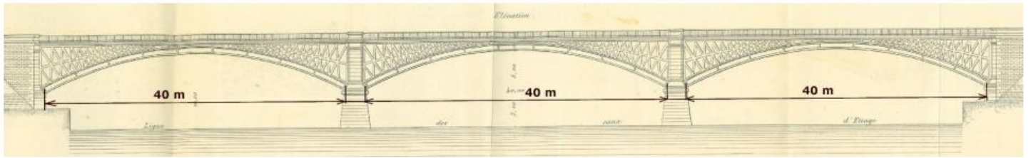
Fig. 1 : Le pont en fonte d'Andenne, projet et réalisation de M. Mouton
